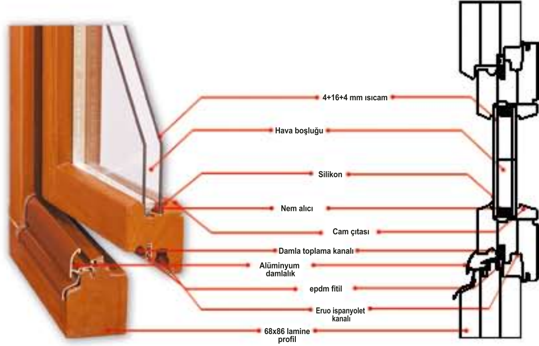
AHŞAP PENCERE KESİTİ
